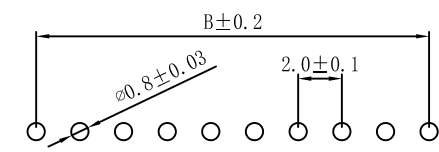
P.C.B LAYOUT
